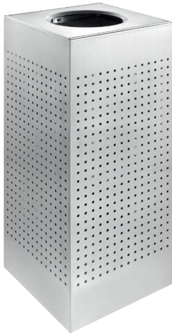
► EK94927 A: L300×W300×H680mm B: L400×W400×H760mm C: L275×W275×H680mm
